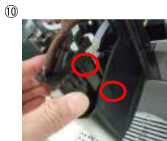
⑩ 抽出口ホルダーと抽出口の○の部分 を合わせるようにします。 (注) セットする際、チューブが折れ曲が らないように注意します。
